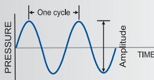
Fig 1-2. Amplitude
